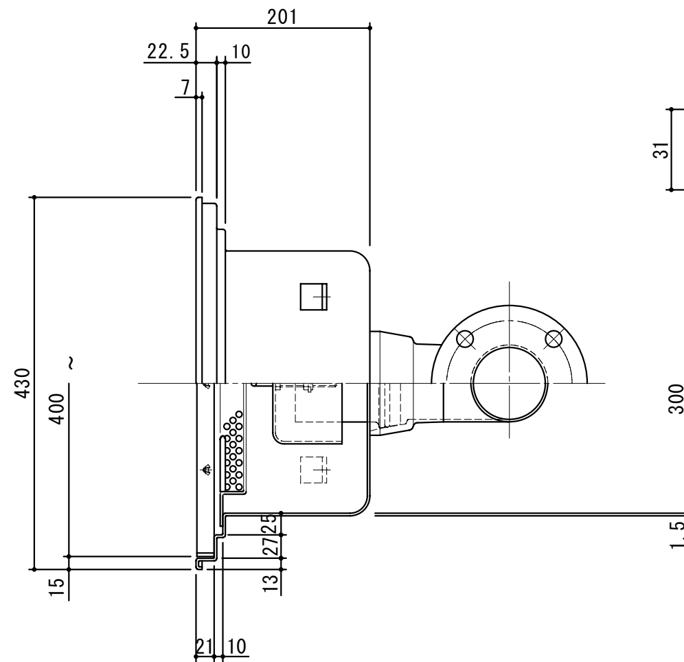
A-A 断面図 S=1:2
