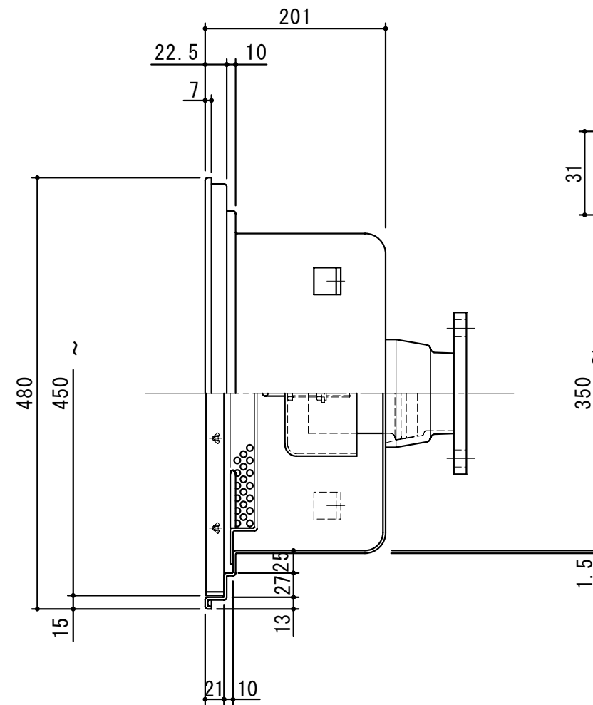
A-A 断面図 S=1:2
