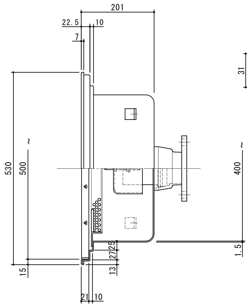
A-A 断面図 S=1:2
