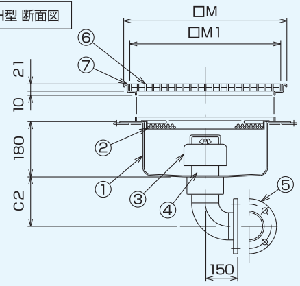
構造図
