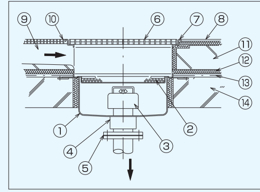
SHB型標準取付図
