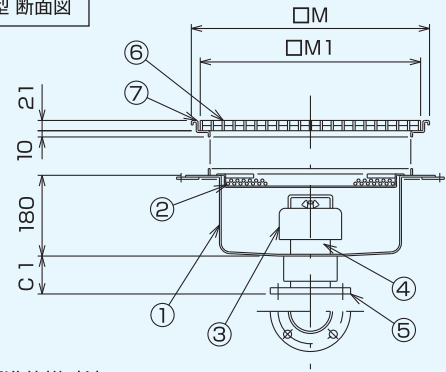
V型断面図
