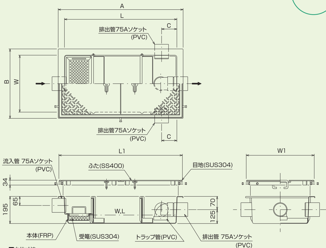
構造図
